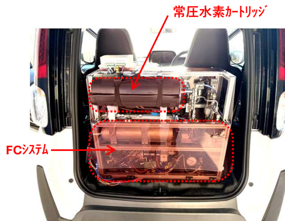
中部電力様向け超小型モビリティ (ベース車：トヨタC+Pod)
